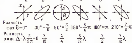
Рис. 2. Примеры различных поляризаций светового луча (траектории конца электрического вектора E в к.-л. одной точке луча) при различных разностях фаз между взаимно перпендикулярными компонентами E x и E y . Плоскость рисунков перпендикулярна направлению распространения света; а и д — линейные поляризации; в — правая круговая поляризация; б, г и е — эллиптические поляризации различной ориентации. Приведённые рисунки соответствуют положительным разностям фаз \delta (опережению вертикальных колебаний по сравнению с горизонтальными). \lambda — длина волны света.
